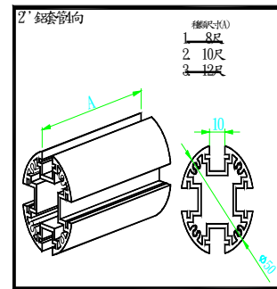
B2072C 2" 鋁套管4向10尺銀
