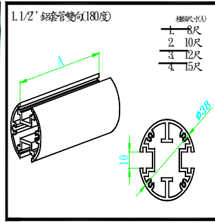
B2022C 1.1/2" 鋁套管雙向(180度)10尺銀
