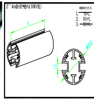
B2042C 2" 鋁套管雙向10尺(180度)銀 B2052C 2" 鋁套管雙向10尺(90度)銀
