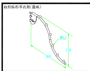
D0030C 柱形弧形吊衣架(圓珠)銀
