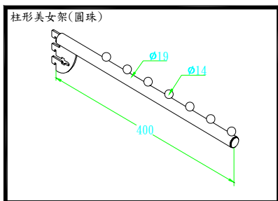
D0130C 柱形美女架銀 圓珠
