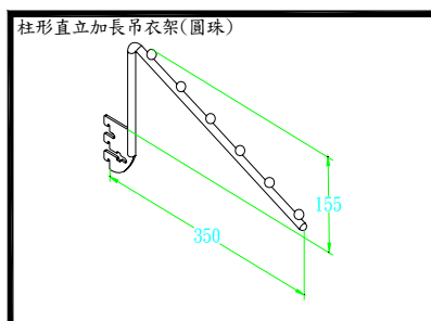
D0050C 柱形直立加長吊衣架銀(圓珠)
