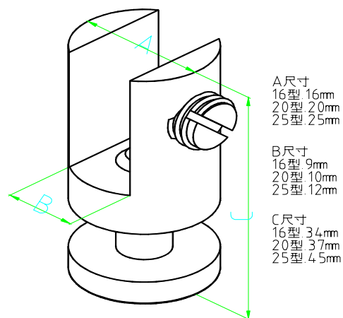
J0060G 16型層止玻璃夾單金 J0070G 20型層止玻璃夾單金 J0081G 25型層止玻璃夾單金
