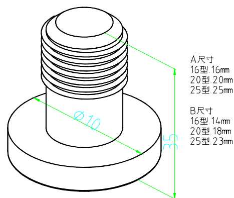
J0061G 16型層止玻璃夾頭金 J0071G 20型層止玻璃夾頭金 J0080G 25型層止玻璃夾頭金
