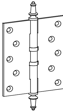
L30073 皇冠頭銅培林 5" * 4" * 3.2mm
