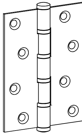
L30040 平頭白鐵培林 - 毛絲面 4"*3"*2.0mm
