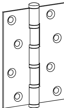
L30041 平頭白鐵培林 - 毛絲面 4"*3"*3.0mm
