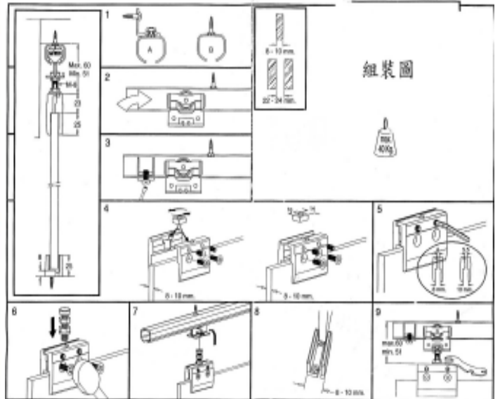
P10010 玻璃懸吊系統SV-40 公斤毛絲 P10002 玻璃懸吊系統軌道-2.5M 毛絲
