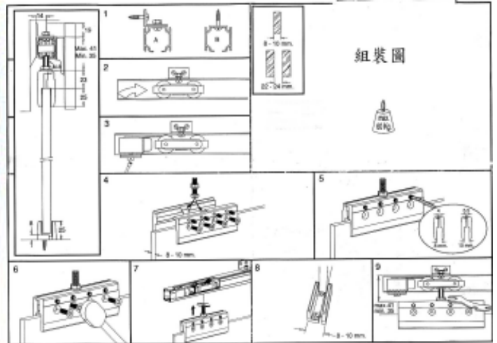
P10020F 玻璃懸吊系統 SV-60F 60 公斤 P10001 玻璃懸吊系統軌道 -2.5M 鋁
