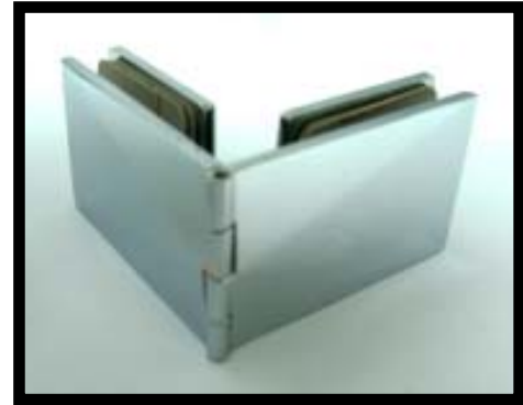
編號：RG0016CH, SC 外銷大鑽石玻對玻璃鉸鍊 產品色澤：FIN(亮銀CH、霧銀SC) PAT：77768(專利字號) 產品用途：玻璃、木工通用 工業技術研究院/ 系統與航太技術發展中心測試 (工服編號：T2004303A0)
